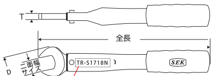
型式 TR-S1718N (締めトルク値 18N・m) (二面幅サイズ)
